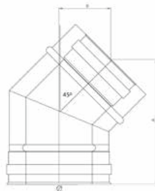
ELBOW 45°
