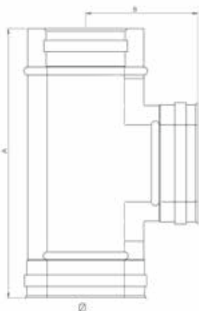
TEE 90°
