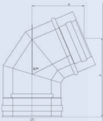
ELBOW 67°
