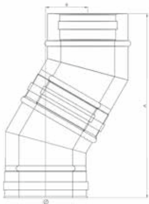
ΓΩΝΙΑ 30°
