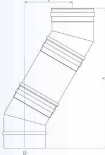
ΓΩΝΙΑ 30° ΜΕ ΚΟΜΜΑΤΙ 0.25m
