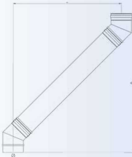
ΓΩΝΙΑ 45° ΜΕ ΚΟΜΜΑΤΙ 1m
