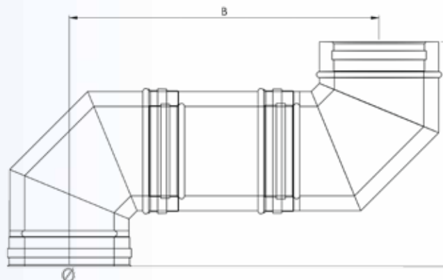
ΓΩΝΙΑ 90° ΜΕ ΚΟΜΜΑΤΙ 0.25m
