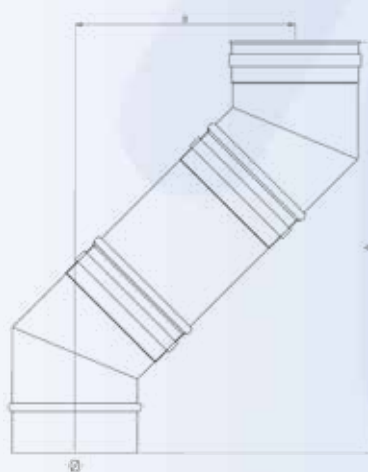
ΓΩΝΙΑ 45° ΜΕ ΚΟΜΜΑΤΙ 0.25m
