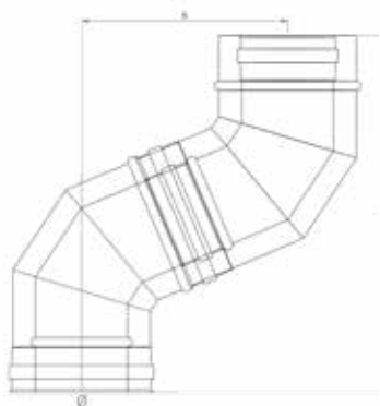
ΓΩΝΙΑ 67°
