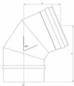
ΓΩΝΙΑ 67°
