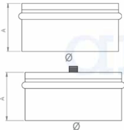
ΤΑΠΑ ΑΡΣ.
