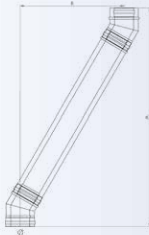
ΓΩΝΙΑ 30° ΜΕ ΚΟΜΜΑΤΙ 1m
