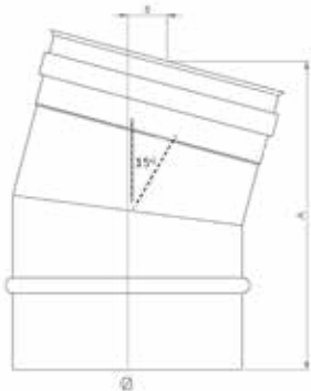
ΓΩΝΙΑ 15°
