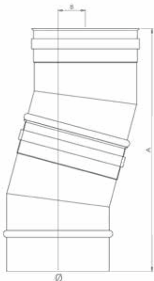
ΓΩΝΙΑ 15°
