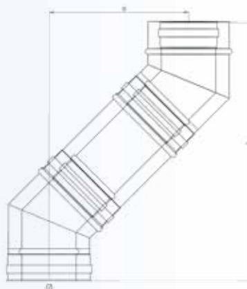
ΓΩΝΙΑ 45° ΜΕ ΚΟΜΜΑΤΙ 0.25m
