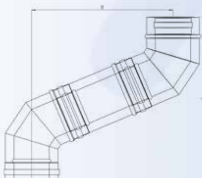
ΓΩΝΙΑ 67° ΜΕ ΚΟΜΜΑΤΙ 0.25m
