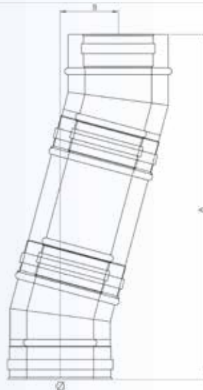
ΓΩΝΙΑ 15° ΜΕ ΚΟΜΜΑΤΙ 0.25m
