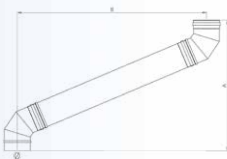
ΓΩΝΙΑ 67° ΜΕ ΚΟΜΜΑΤΙ 1m
