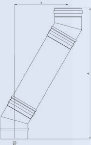
ΓΩΝΙΑ 30° ΜΕ ΚΟΜΜΑΤΙ 0.50m
