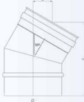
ΓΩΝΙΑ 30°
