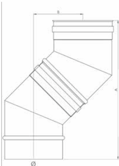
ΓΩΝΙΑ 45°
