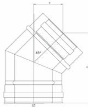
ΓΩΝΙΑ 45°
