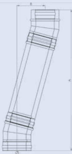
ΓΩΝΙΑ 15° ΜΕ ΚΟΜΜΑΤΙ 0.50m
