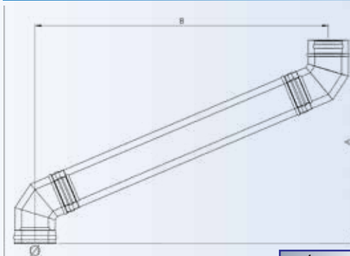
ΓΩΝΙΑ 67° ΜΕ ΚΟΜΜΑΤΙ 1m
